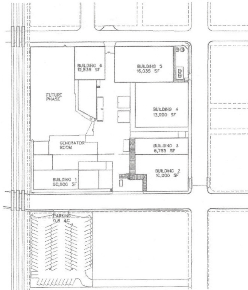
1:1000 SITE PLAN
